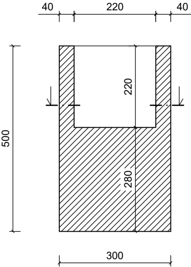
VERTIKALNI PRESEK:
