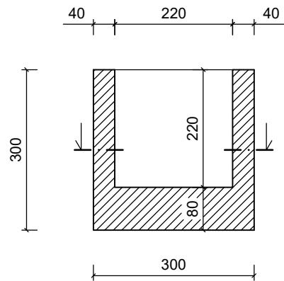
VERTIKALNI PRESEK:
