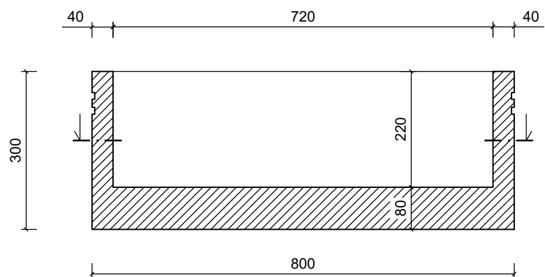
VERTIKALNI PRESEK:
