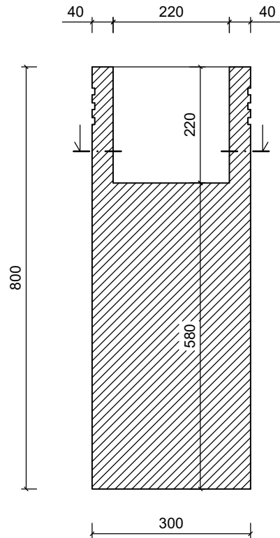
VERTIKALNI PRESEK:
